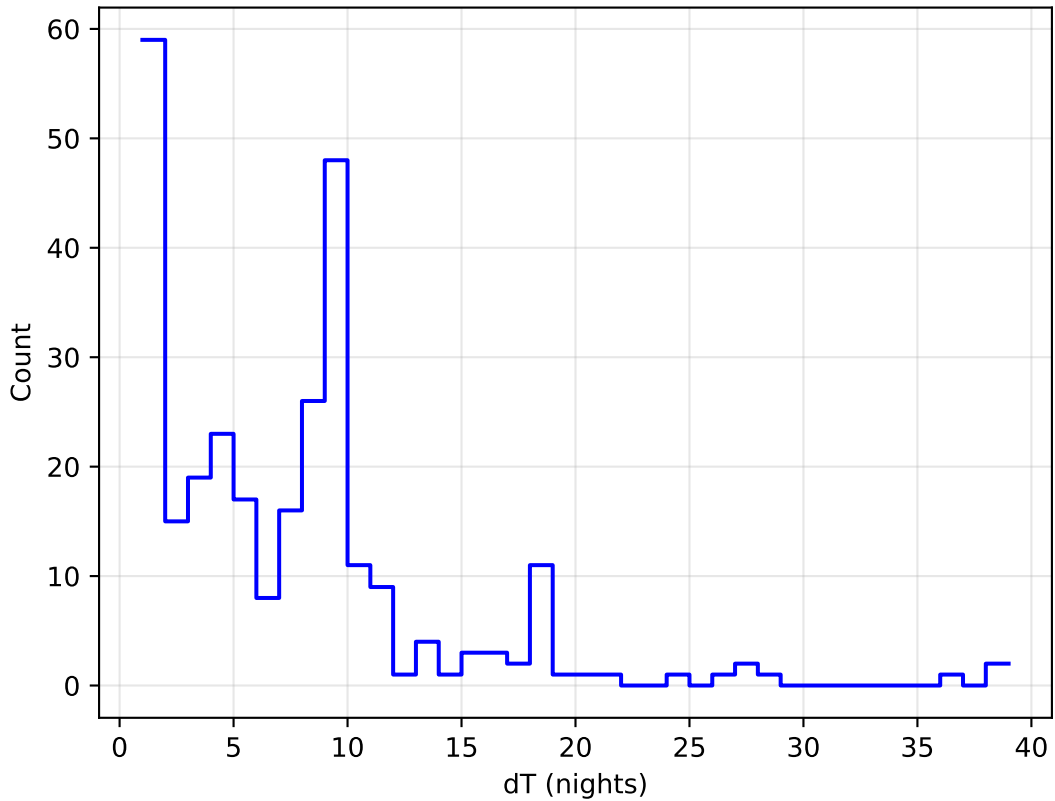
weather_cloudso16v3.4_10yrs all bands: DD:ELAISS1 Delta Nights Histogram
