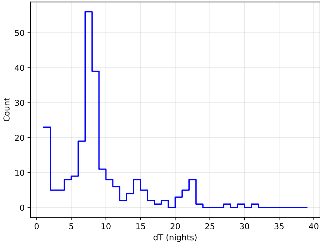
weather_cloudso16v3.4_10yrs all bands: DD:EDFS Delta Nights Histogram
