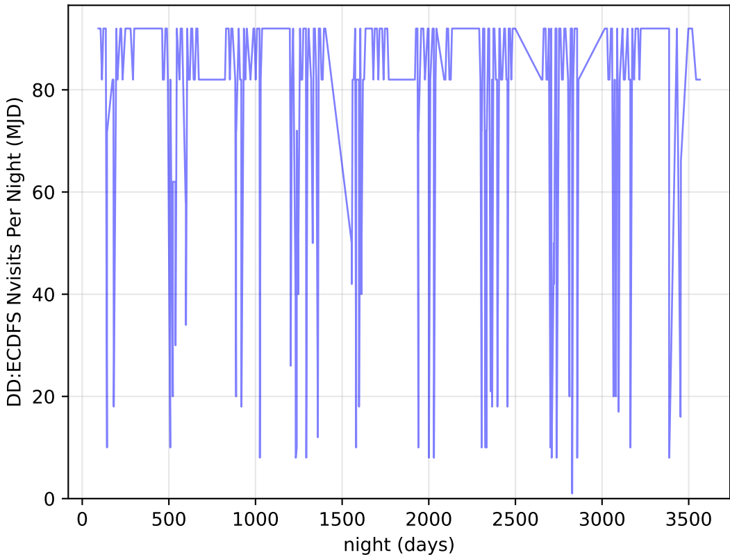
weather_cloudso16v3.4_10yrs all bands: DD:ECDFS Nvisits Per Night
