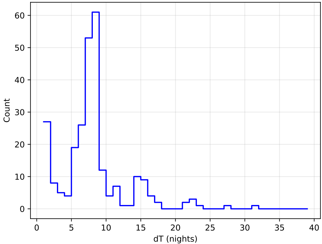
weather_cloudso16v3.4_10yrs all bands: DD:ECDFS Delta Nights Histogram
