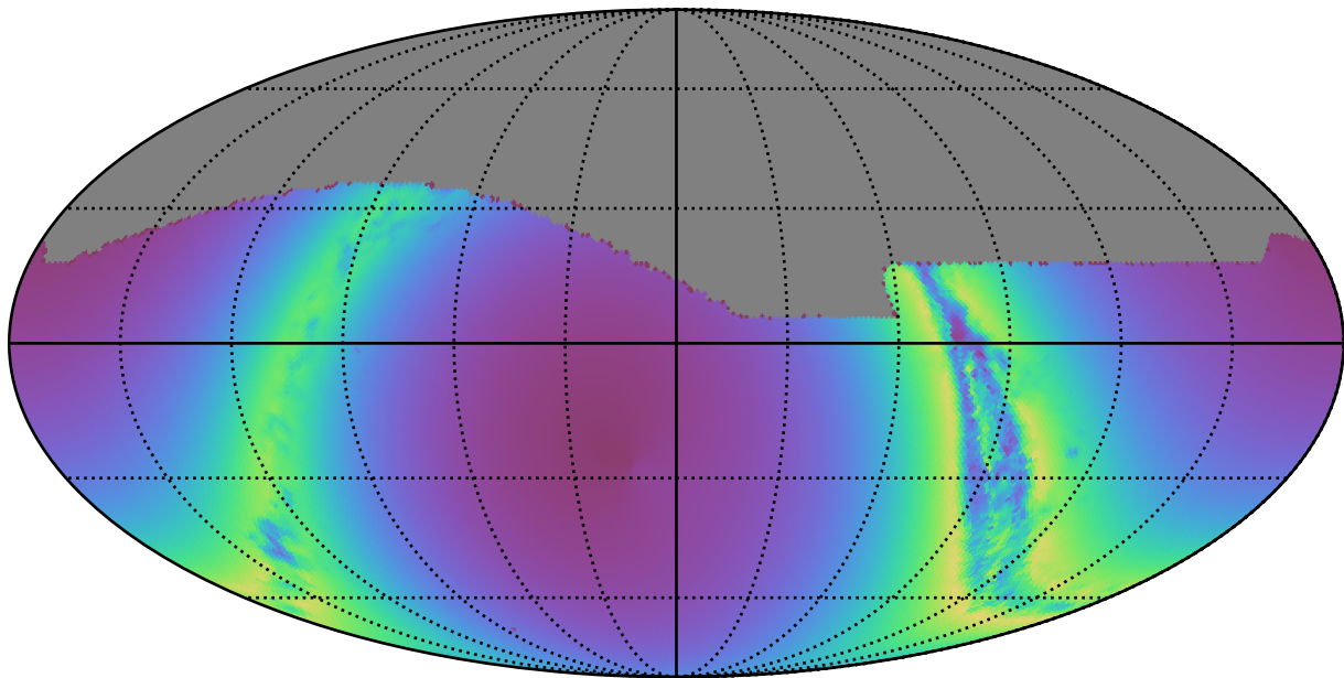
weather_cloudso14v3.4_10yrs : young_stars
