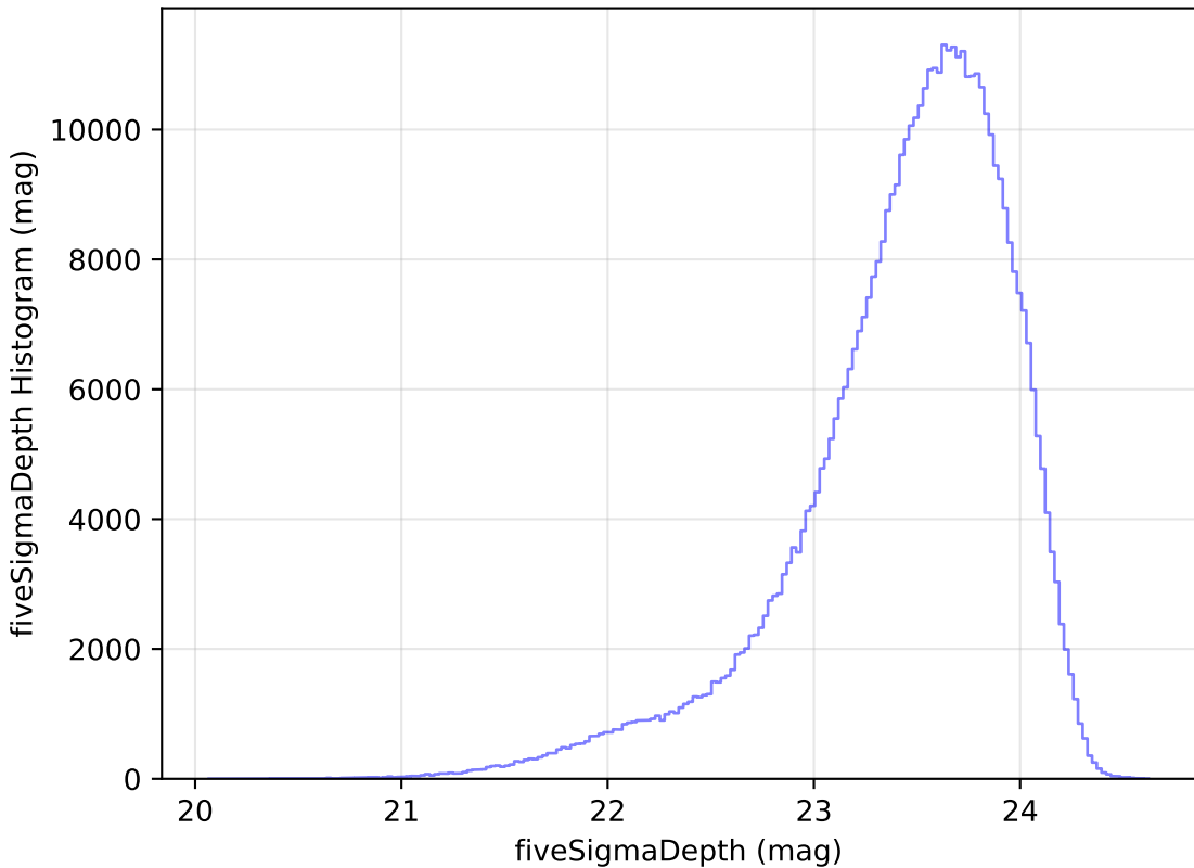
weather_cloudso14v3.4_10yrs i: fiveSigmaDepth Histogram
