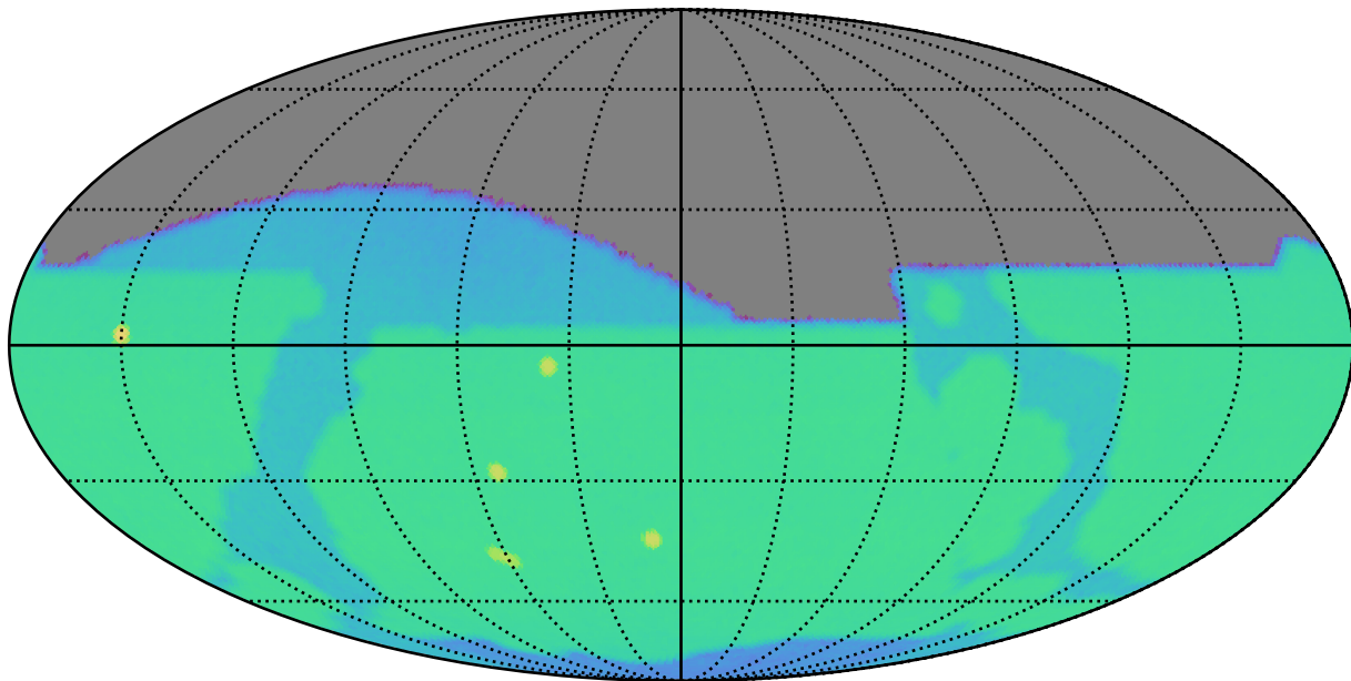
weather_cloudso14v3.4_10yrs i: SurfaceBrightLimit
