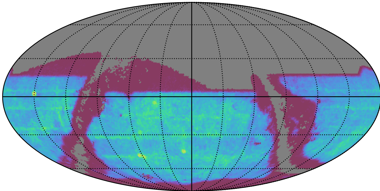
weather_cloudso14v3.4_10yrs : SNSLMetric
