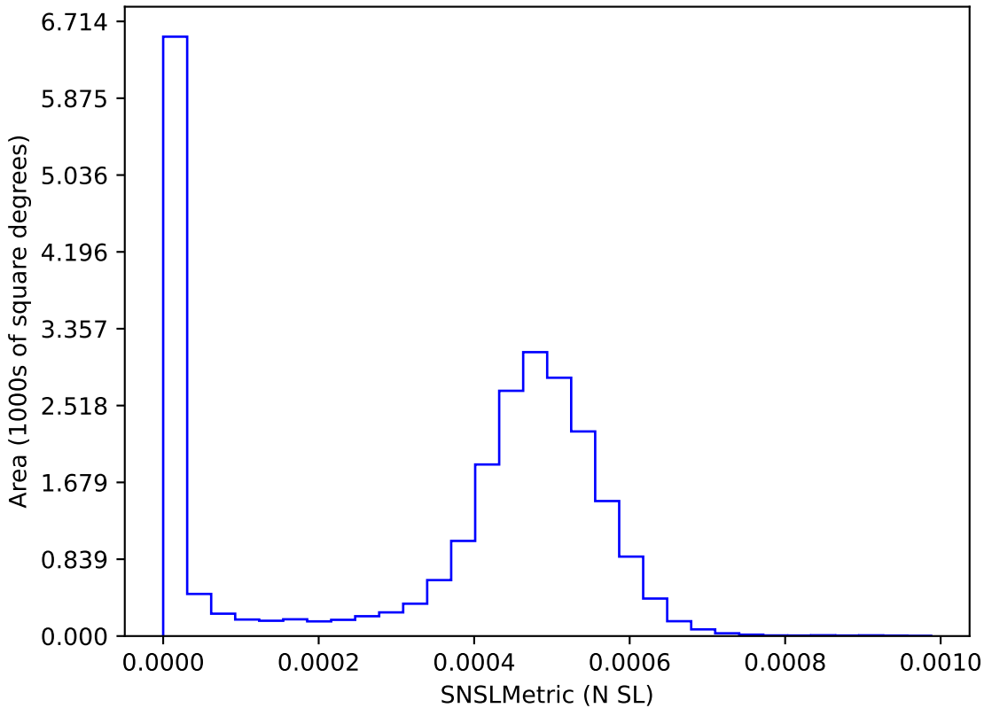
weather_cloudso14v3.4_10yrs : SNSLMetric
