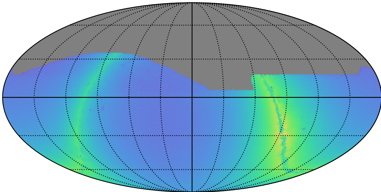
weather_cloudso14v3.4_10yrs z: Nstars_no_crowding
