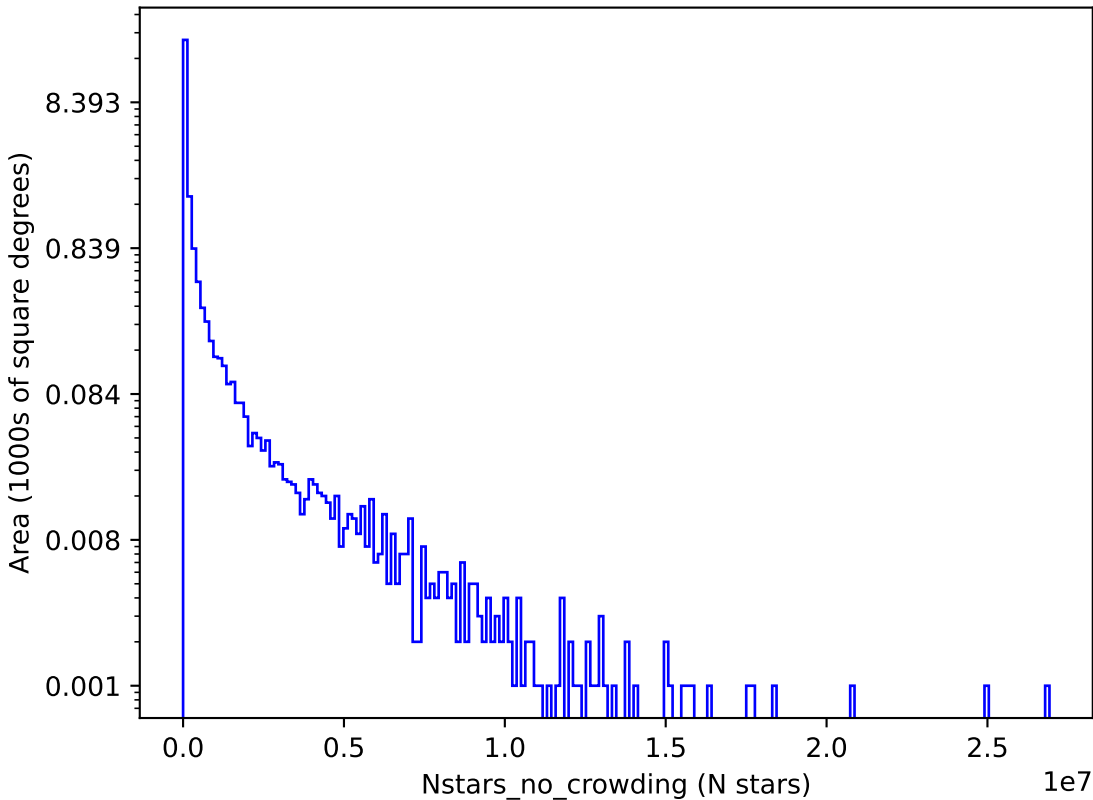
weather_cloudso14v3.4_10yrs z: Nstars_no_crowding
