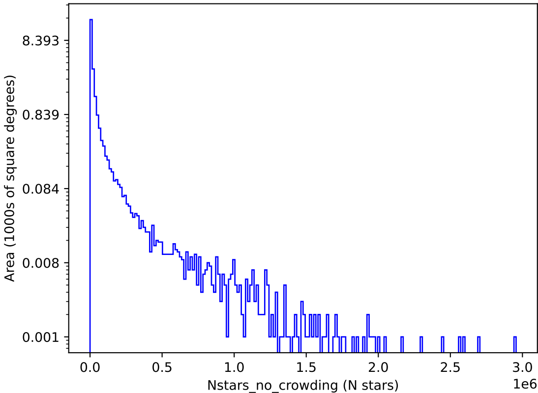
weather_cloudso14v3.4_10yrs u: Nstars_no_crowding
