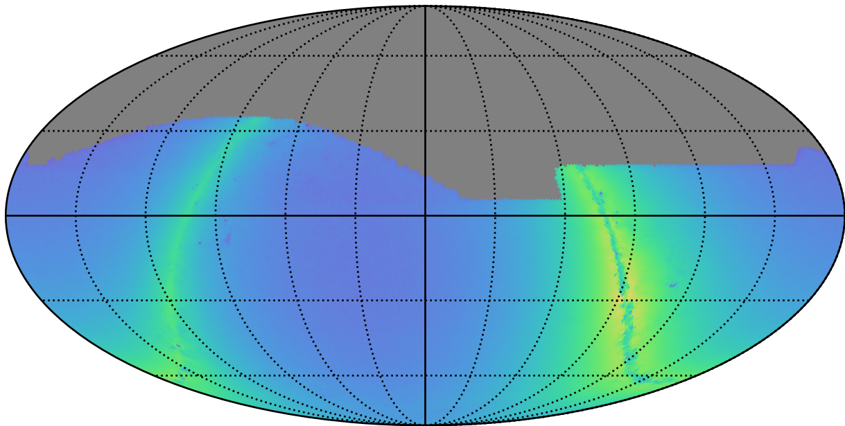
weather_cloudso14v3.4_10yrs i: Nstars_no_crowding
