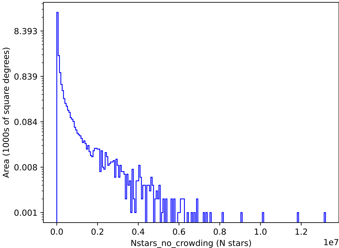
weather_cloudso14v3.4_10yrs g: Nstars_no_crowding
