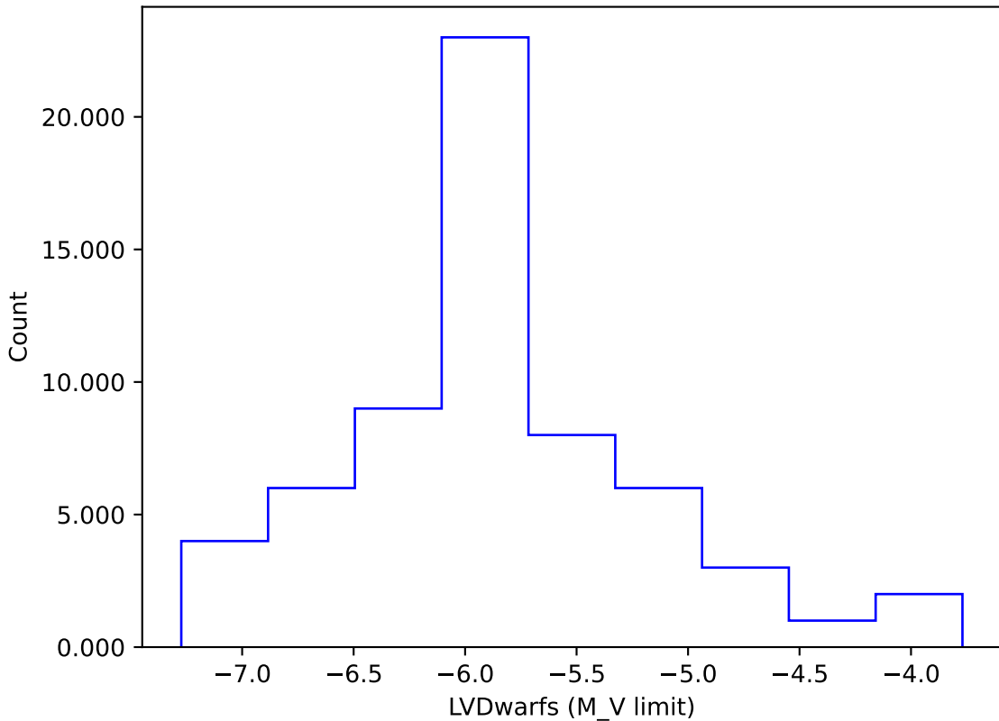
weather_cloudso14v3.4_10yrs gi: LVDwarfs
