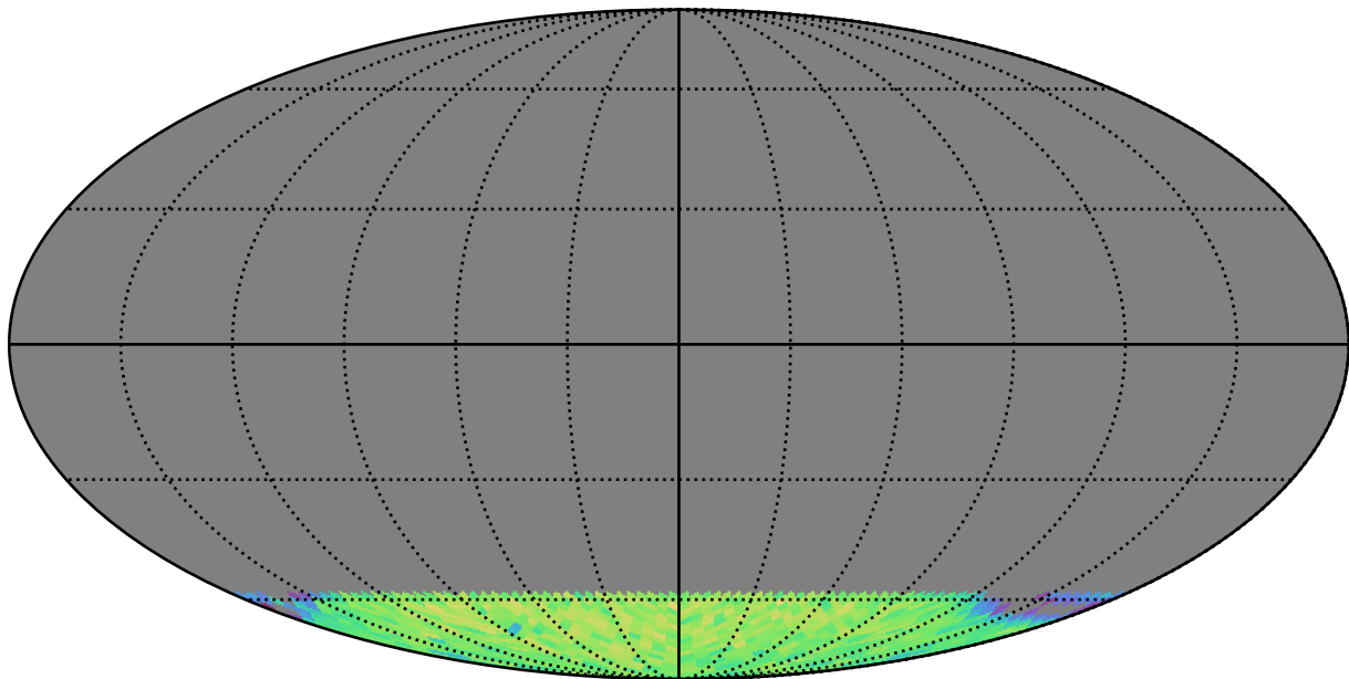
weather_cloudso14v3.4_10yrs gi SCP: LVDwarfs
