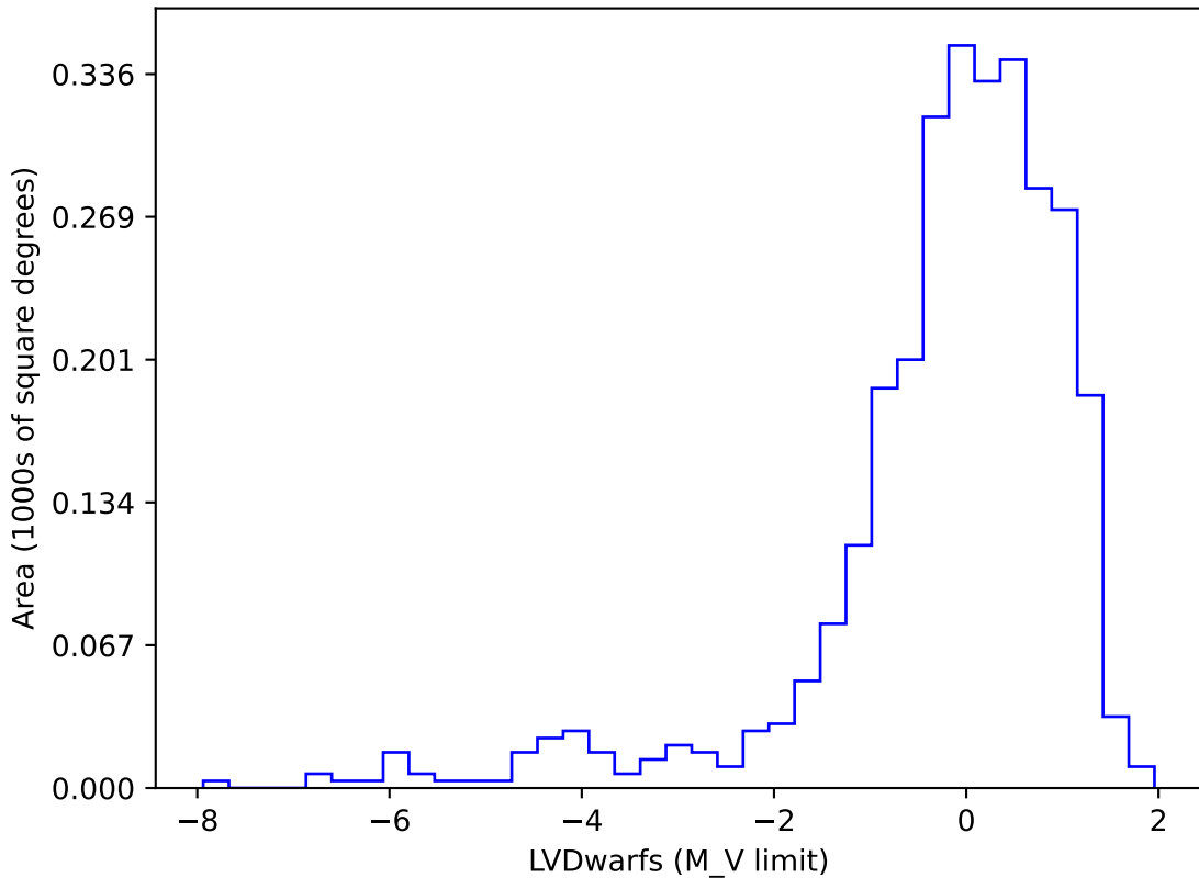
weather_cloudso14v3.4_10yrs gi SCP: LVDwarfs
