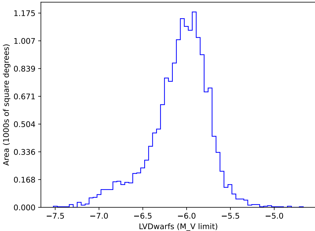
weather_cloudso14v3.4_10yrs gi: LVDwarfs
