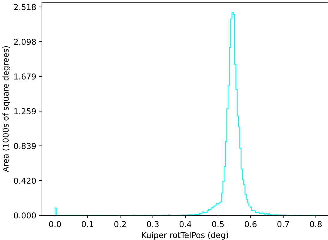
weather_cloudso14v3.4_10yrs u: Kuiper rotTelPos
