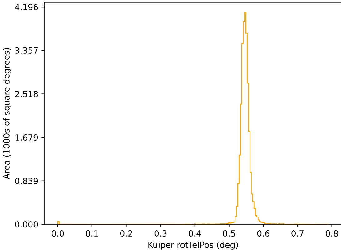
weather_cloudso14v3.4_10yrs r: Kuiper rotTelPos
