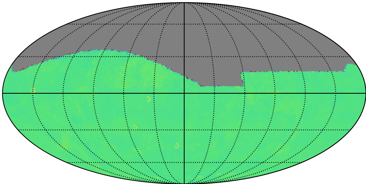
weather_cloudso14v3.4_10yrs i: Kuiper rotTelPos
