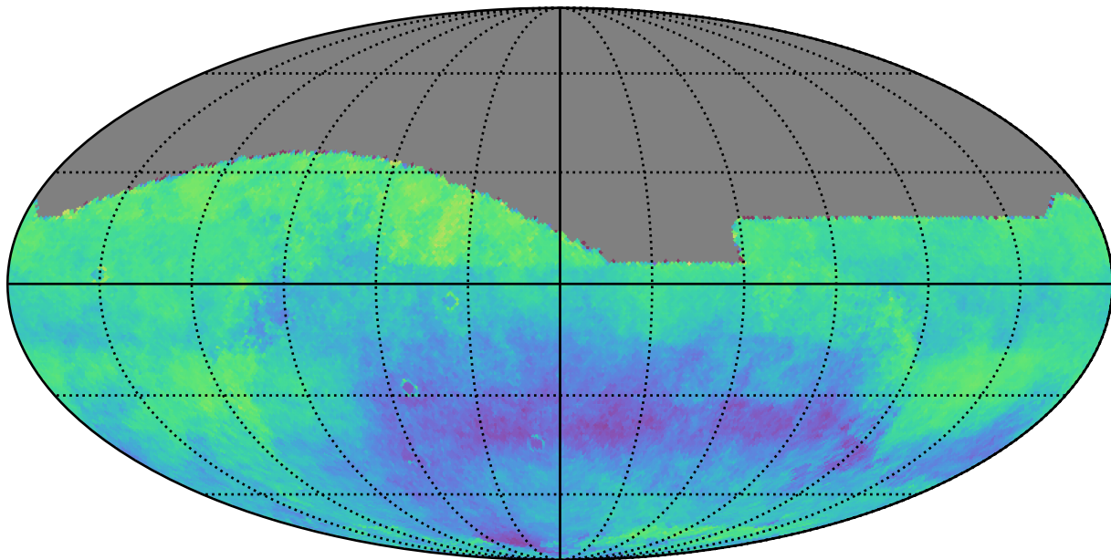
weather_cloudso14v3.4_10yrs z: Kuiper rotSkyPos
