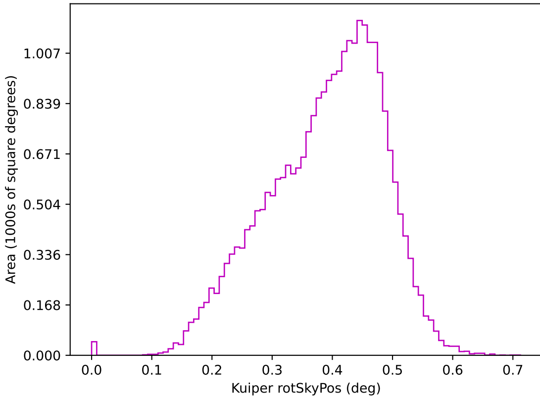
weather_cloudso14v3.4_10yrs z: Kuiper rotSkyPos
