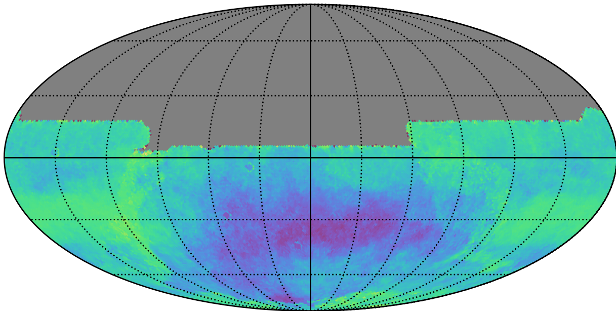
weather_cloudso14v3.4_10yrs y: Kuiper rotSkyPos
