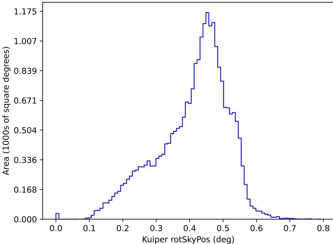
weather_cloudso14v3.4_10yrs y: Kuiper rotSkyPos
