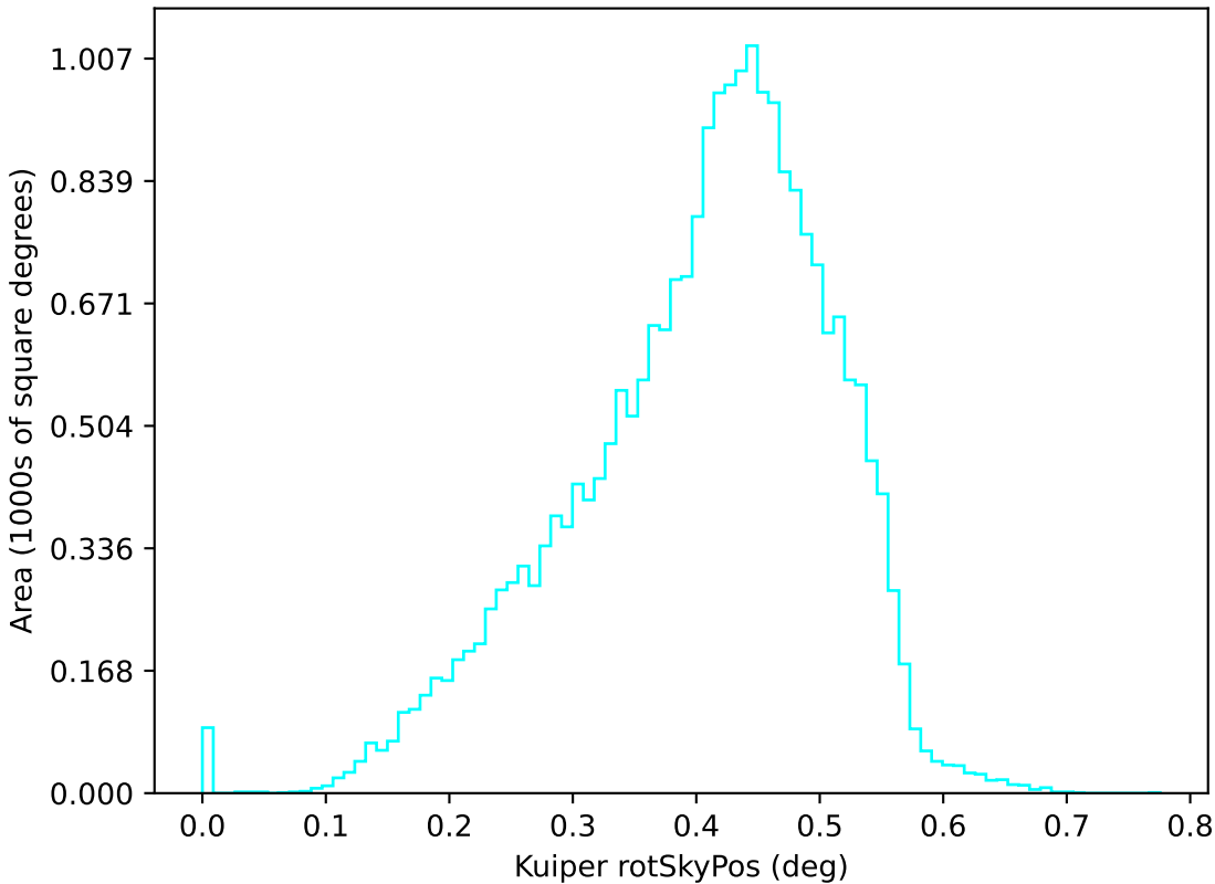
weather_cloudso14v3.4_10yrs u: Kuiper rotSkyPos
