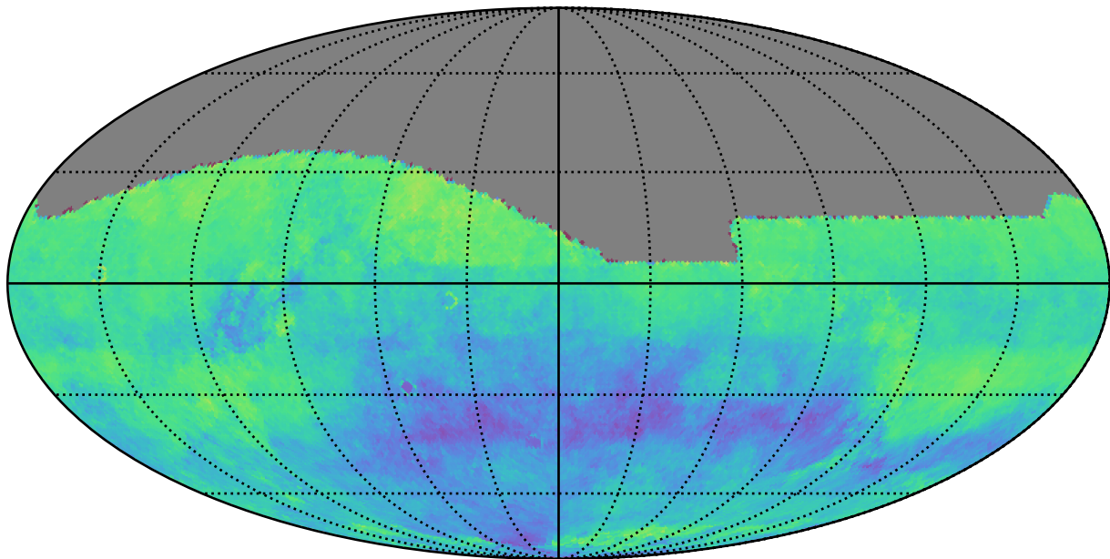
weather_cloudso14v3.4_10yrs i: Kuiper rotSkyPos
