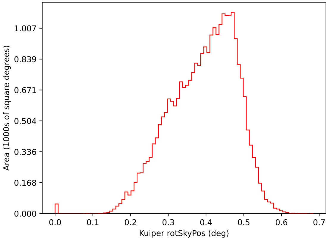
weather_cloudso14v3.4_10yrs i: Kuiper rotSkyPos
