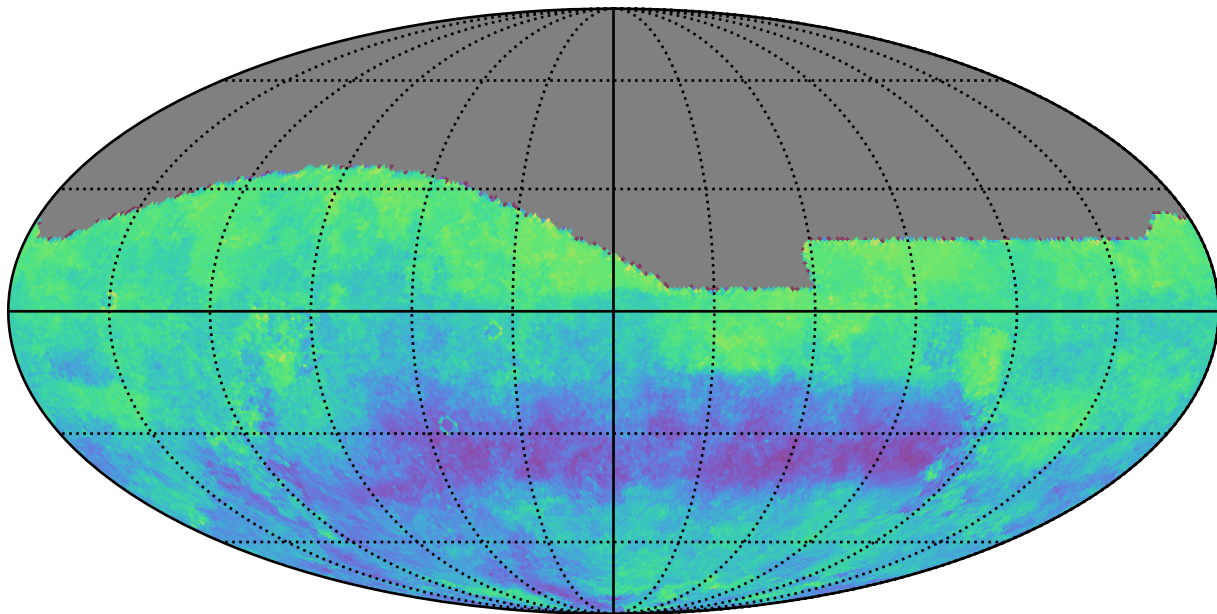
weather_cloudso14v3.4_10yrs g: Kuiper rotSkyPos
