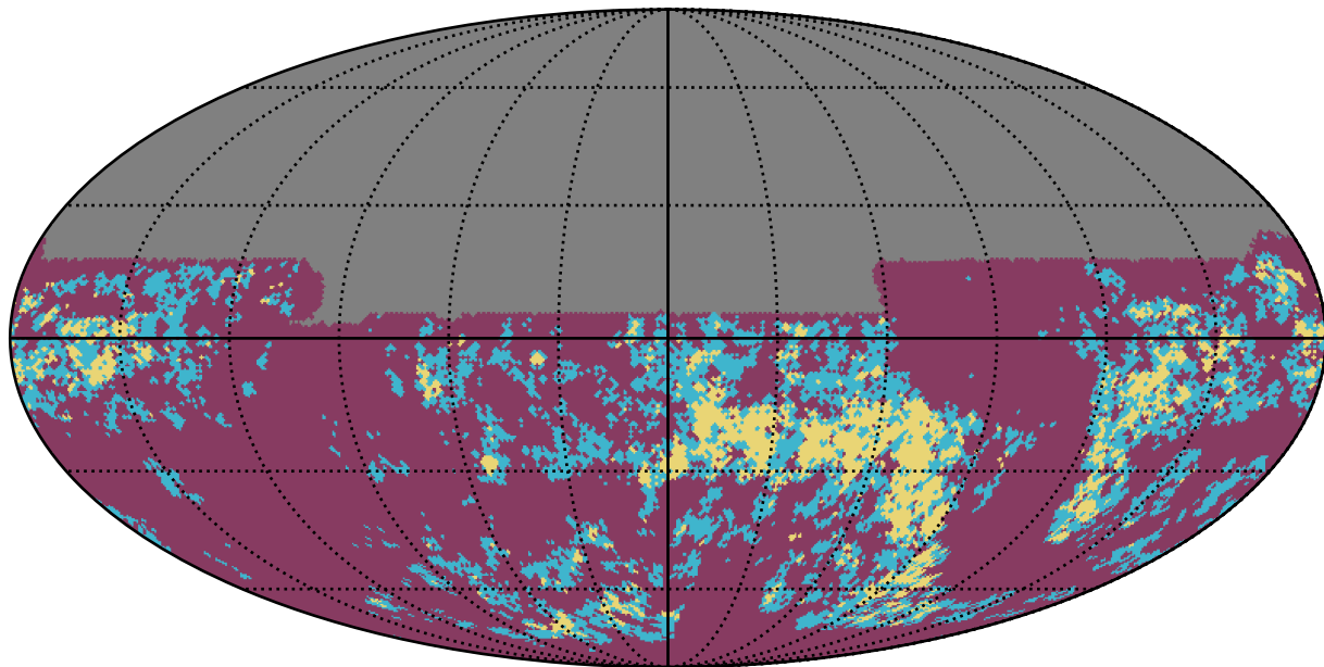
weather_cloudso14v3.4_10yrs y band: Gaps_7hr
