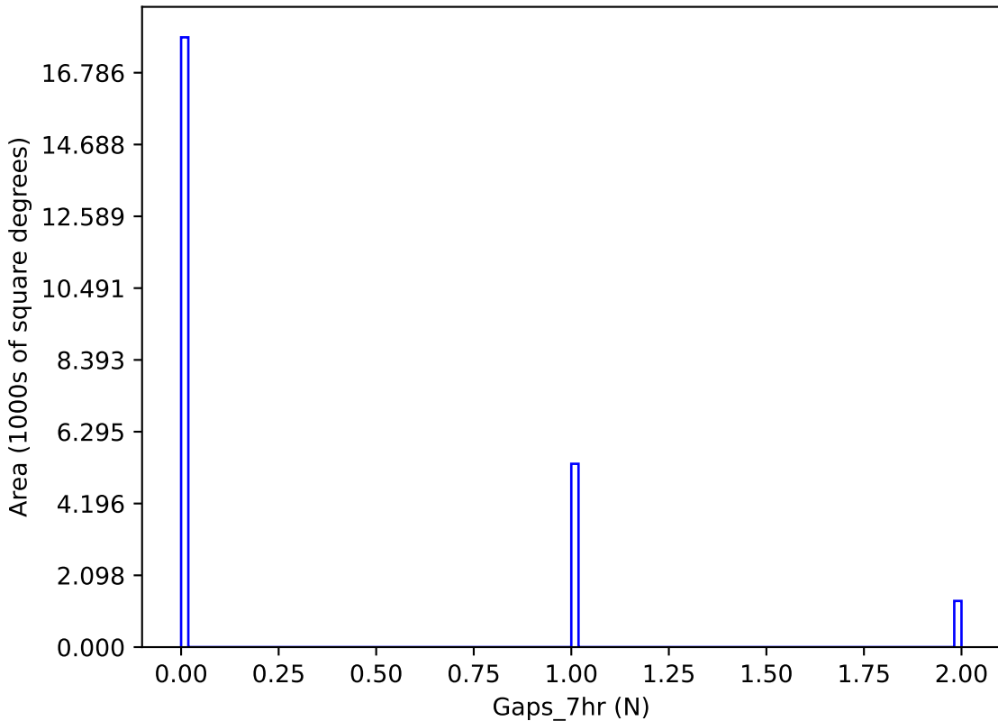
weather_cloudso14v3.4_10yrs y band: Gaps_7hr
