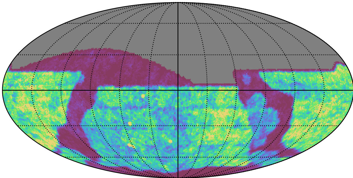
weather_cloudso14v3.4_10yrs z band: Gaps_24hr
