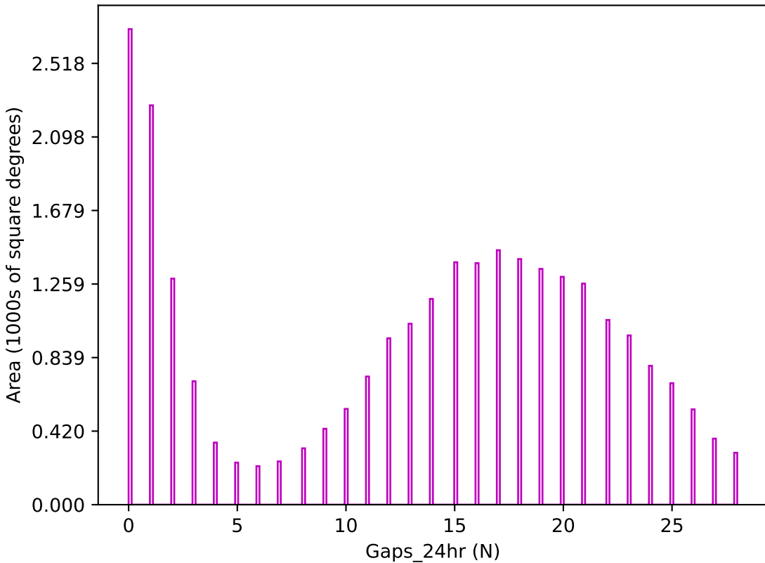
weather_cloudso14v3.4_10yrs z band: Gaps_24hr
