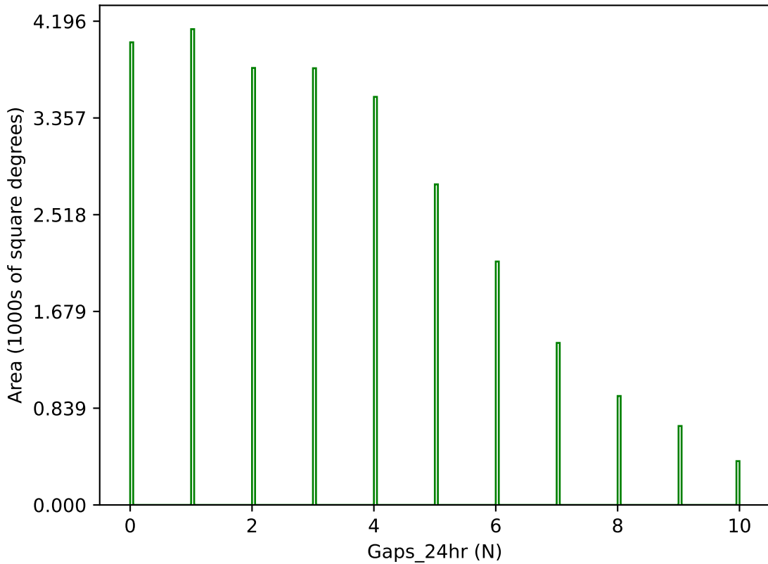
weather_cloudso14v3.4_10yrs g band: Gaps_24hr
