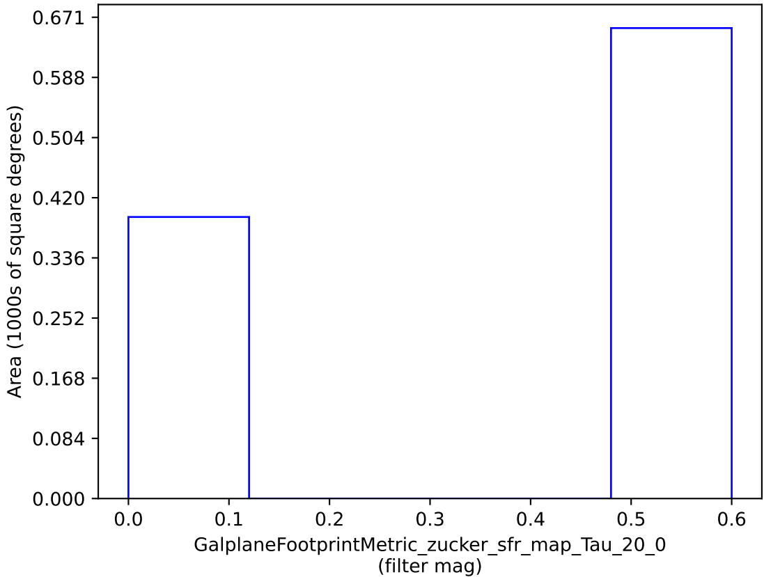
weather_cloudso14v3.4_10yrs : GalplaneFootprintMetric_zucker_sfr_map_Tau_20_0
