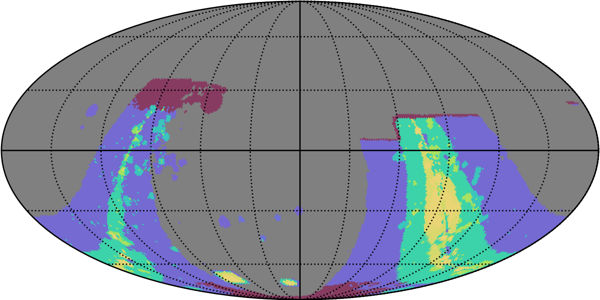
weather_cloudso14v3.4_10yrs : GalplaneFootprintMetric_combined_map_Tau_46_5
