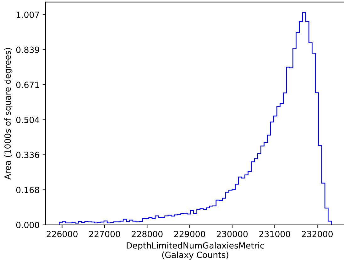
weather_cloudso14v3.4_10yrs i band galaxies non-DD: DepthLimitedNumGalaxiesMetric
