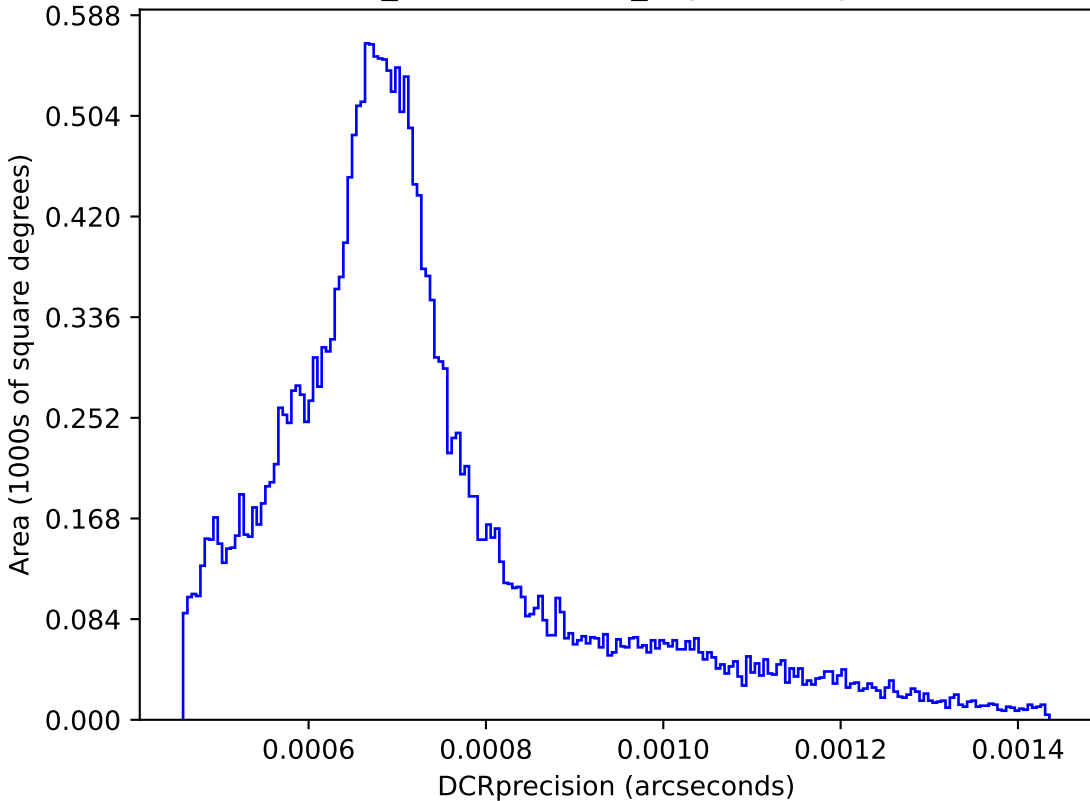
weather_cloudso14v3.4_10yrs : DCRprecision
