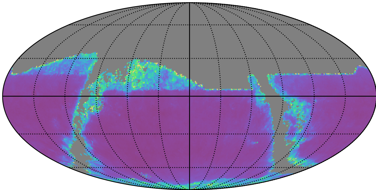
weather_cloudso14v3.4_10yrs z band: AGN SF_uncert
