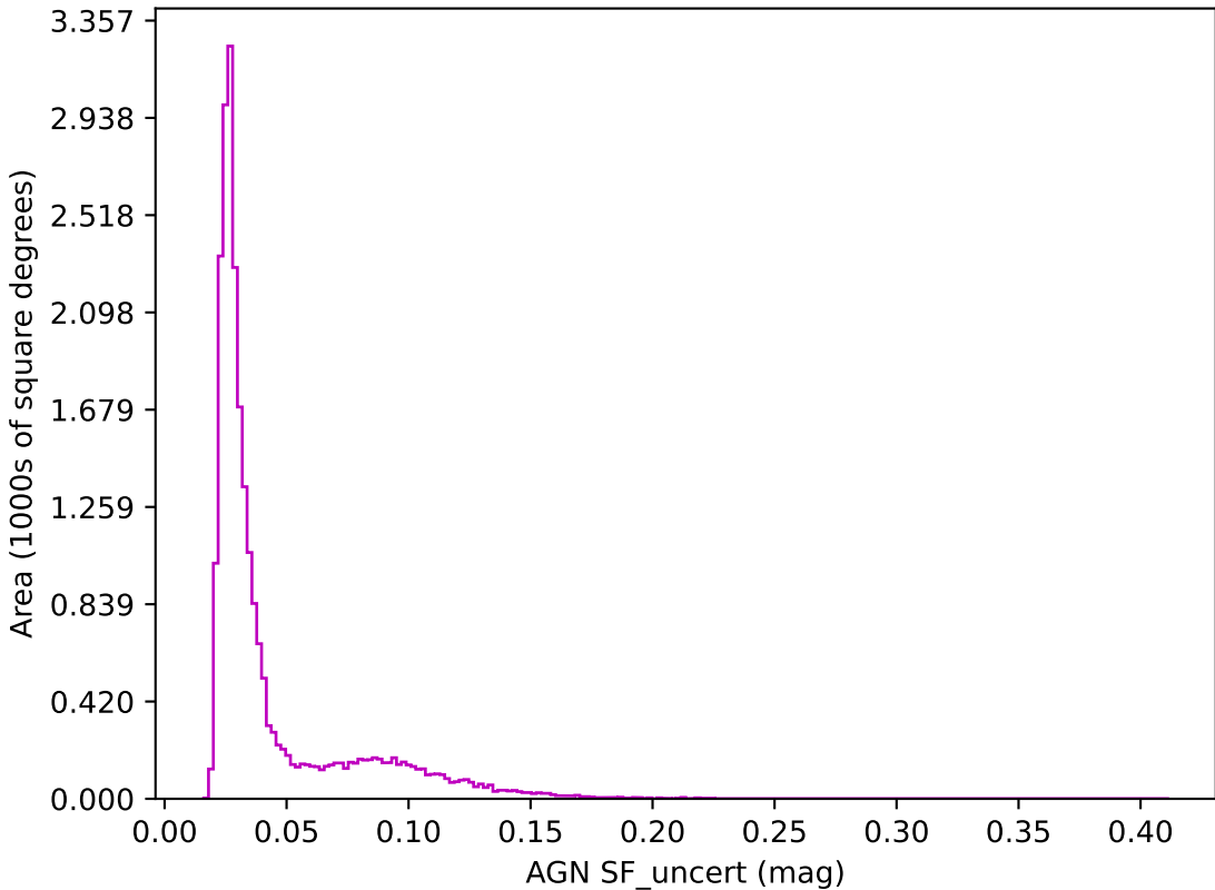
weather_cloudso14v3.4_10yrs z band: AGN SF_uncert
