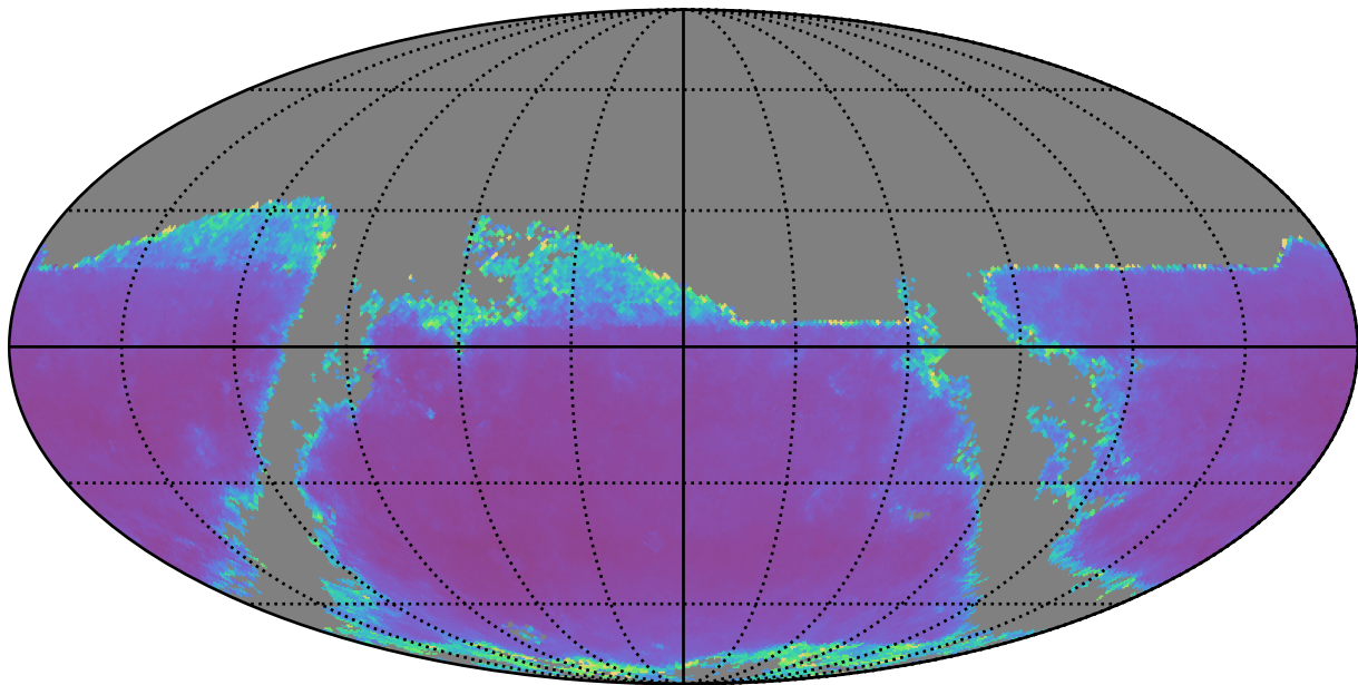
weather_cloudso14v3.4_10yrs r band: AGN SF_uncert
