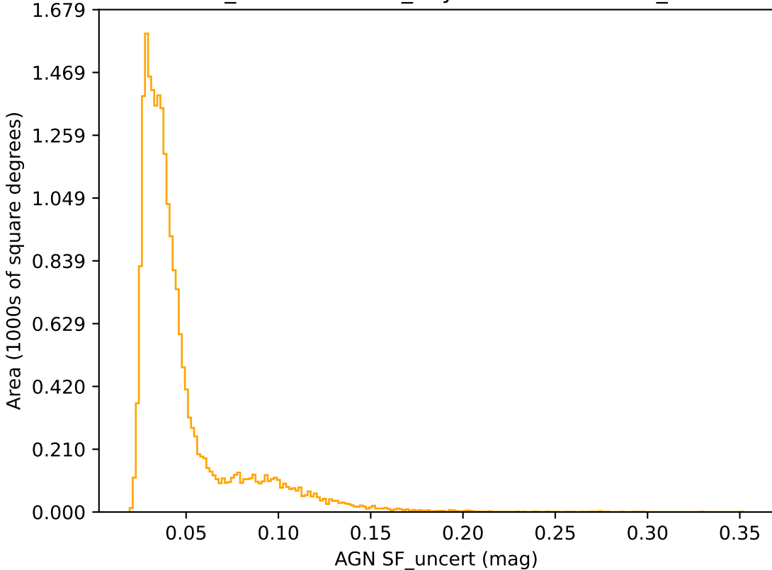
weather_cloudso14v3.4_10yrs r band: AGN SF_uncert
