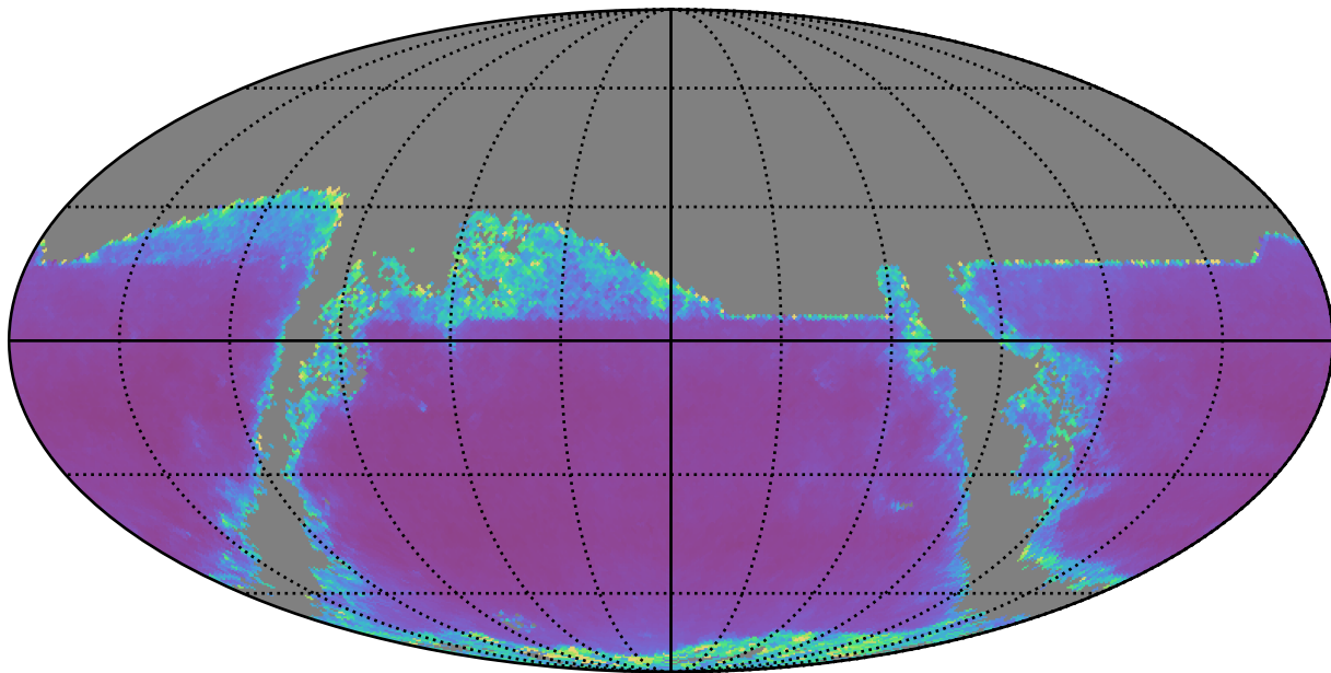
weather_cloudso14v3.4_10yrs i band: AGN SF_uncert
