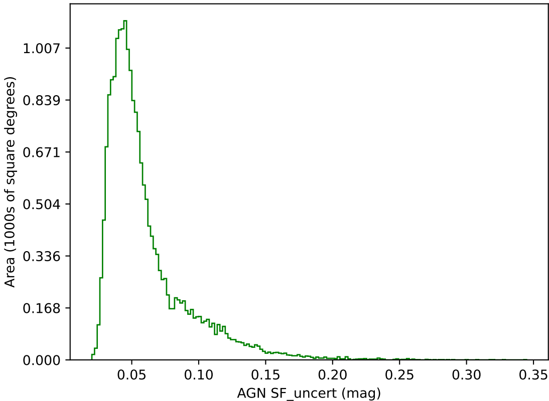
weather_cloudso14v3.4_10yrs g band: AGN SF_uncert
