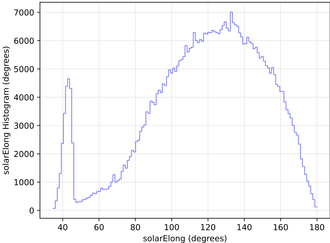
weather_cloudso14v3.4_10yrs WFD z band: solarElong Histogram
