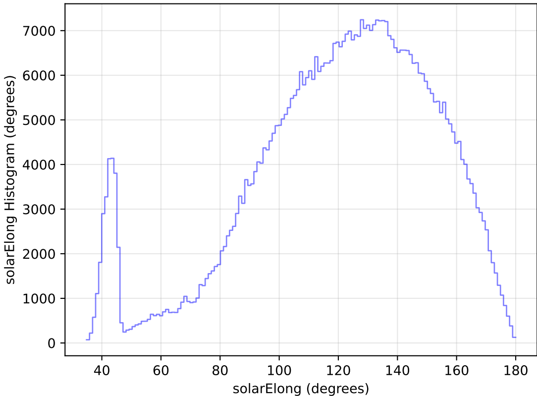
weather_cloudso14v3.4_10yrs WFD i band: solarElong Histogram
