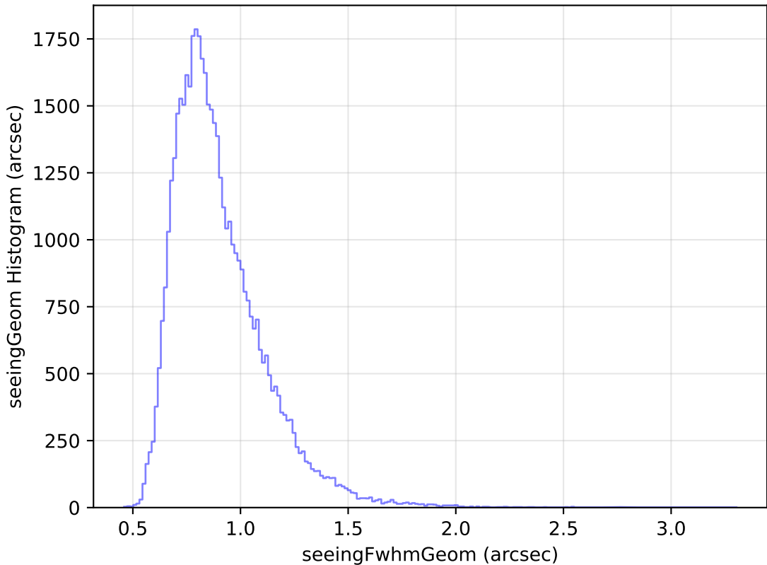
weather_cloudso14v3.4_10yrs Yr 1 y band: seeingGeom Histogram
