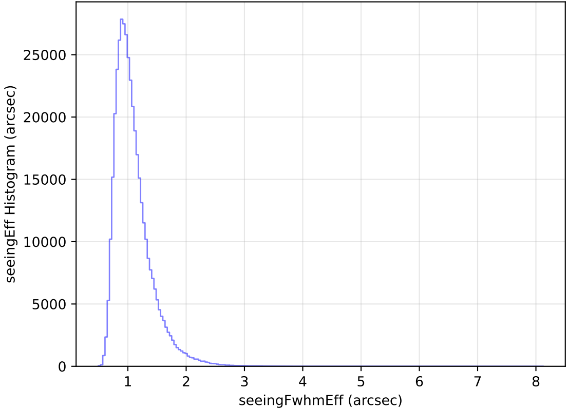
weather_cloudso14v3.4_10yrs WFD y band: seeingEff Histogram
