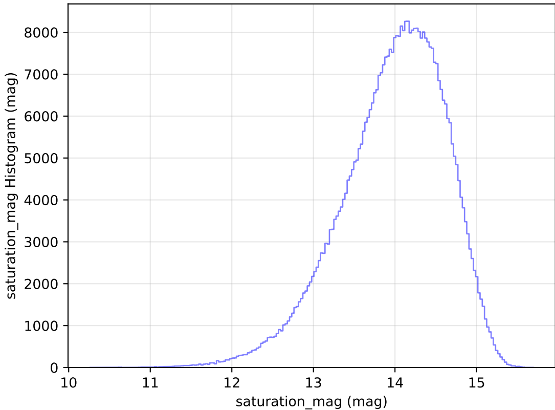
weather_cloudso14v3.4_10yrs WFD z band: saturation_mag Histogram
