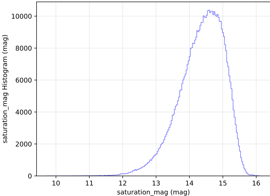
weather_cloudso14v3.4_10yrs WFD i band: saturation_mag Histogram
